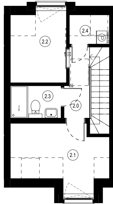
PIĘTRO I
