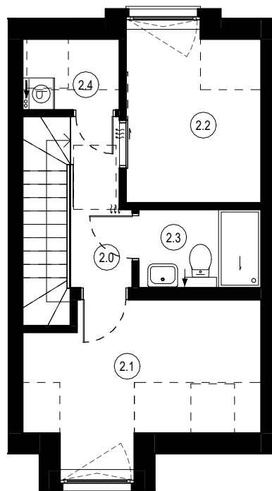
PIĘTRO I
